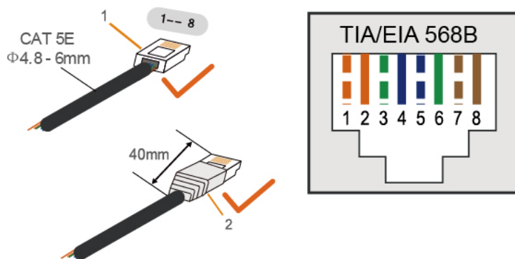
1: Fiche RJ45
